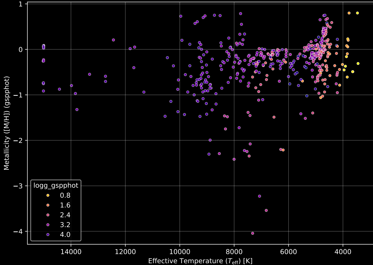
APOGEE DR17 Field: [094+00] Stellar Population Parameters (n= 459)
